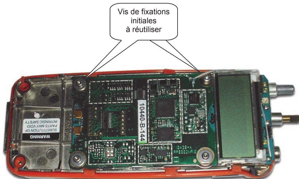
Vue d'intégration sur le châssis du portatif radio
